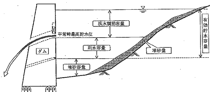
貯水池等の概念図
