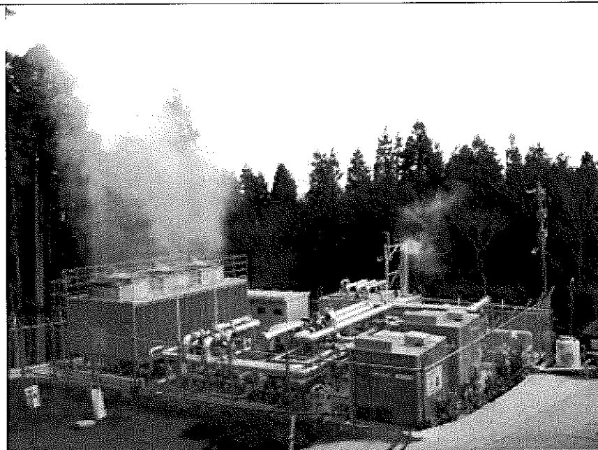
五湯苑地熱発電所の外観。空色の箱が2台のバイナリー発電機
