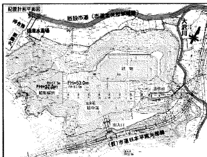
新斎場配置計画平面図 (平成25年9月現在)
