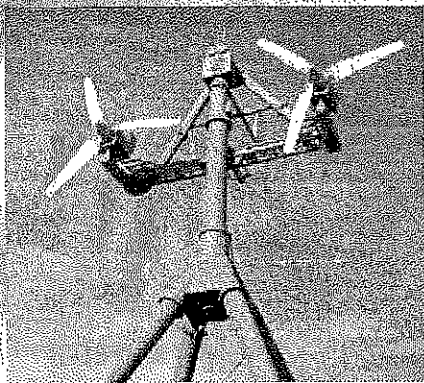
ツインローター型風力発電機
